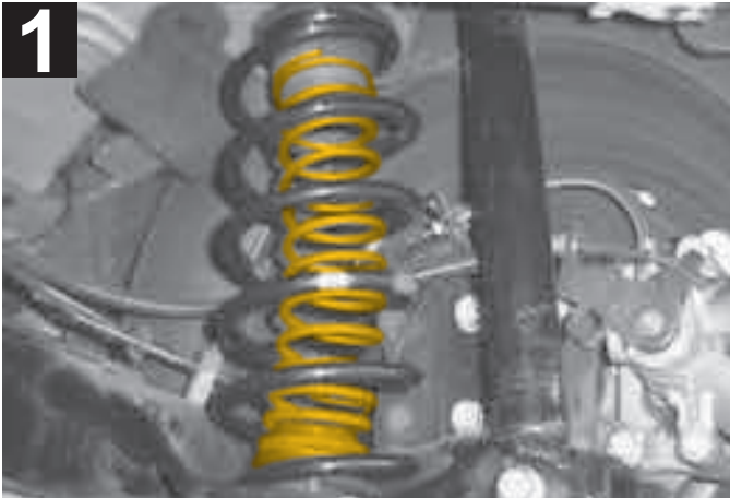
1 Interna al mollone originale Inside the original suspension spring In der Originalfeder - A l'intérieur du ressort existant Al interno muelles originales - In de hoofveer
